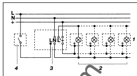
1. Svjetiljka bez postojećeg nulnog vodiča
