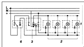
4. Připojení prostřednictvím střídatvého přepínače pro trvalé osvětlení a automatický provoz
