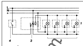
1. Armatur med nolledaren ansluten via sensor.
